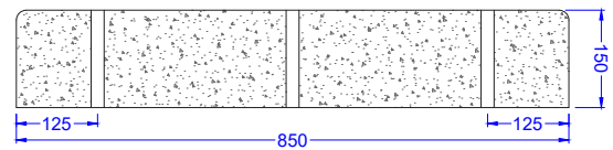
COUPE B-B
